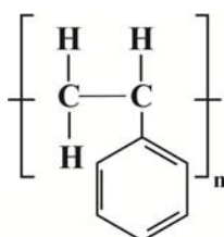
ترکیب (۱)
