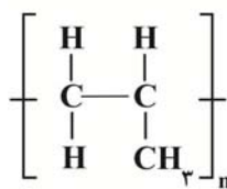
ترکیب (۳)
