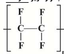
ترکیب (۲)
