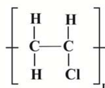
ترکیب (۴)
